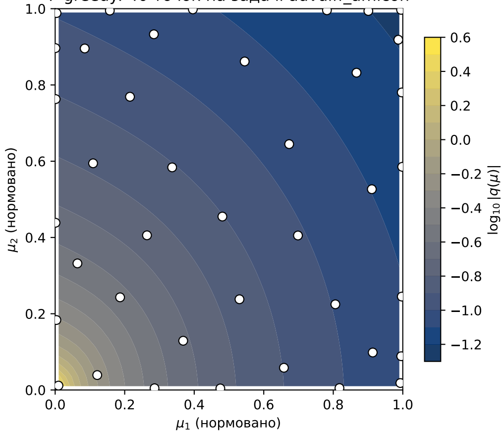
P-greedy: 40 точок на задачі advdiff_amicon
